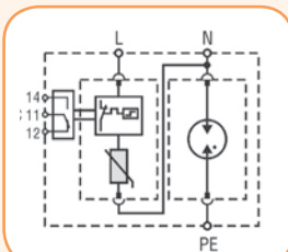
ETIТЕС C EV (1+1) RC
